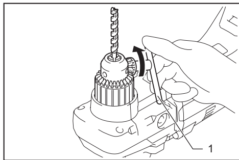
► 1. Chuck key
